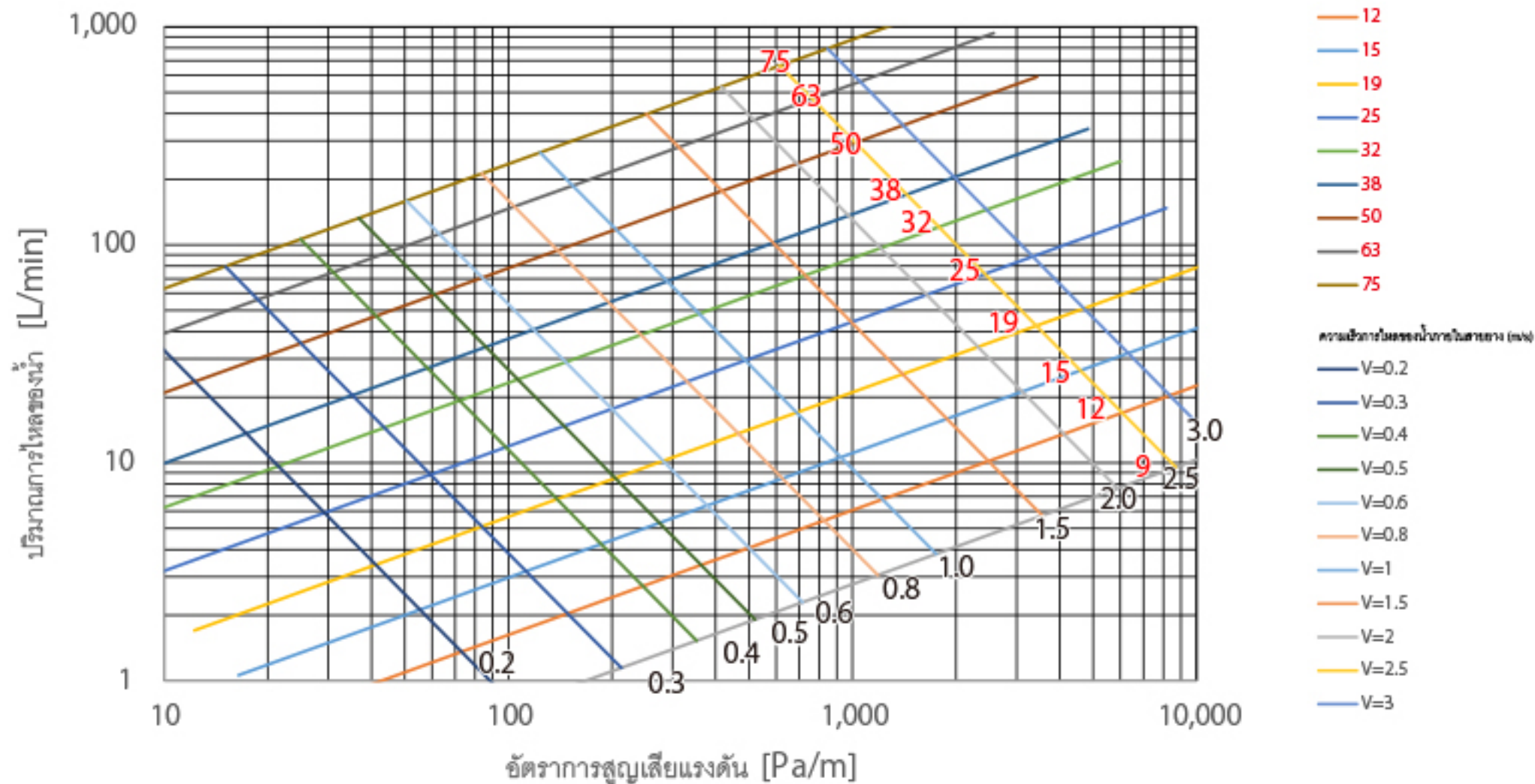
แผนภาพแสดงอัตราการไหลของน้ำ (อุณหภูมิ 25°C)
